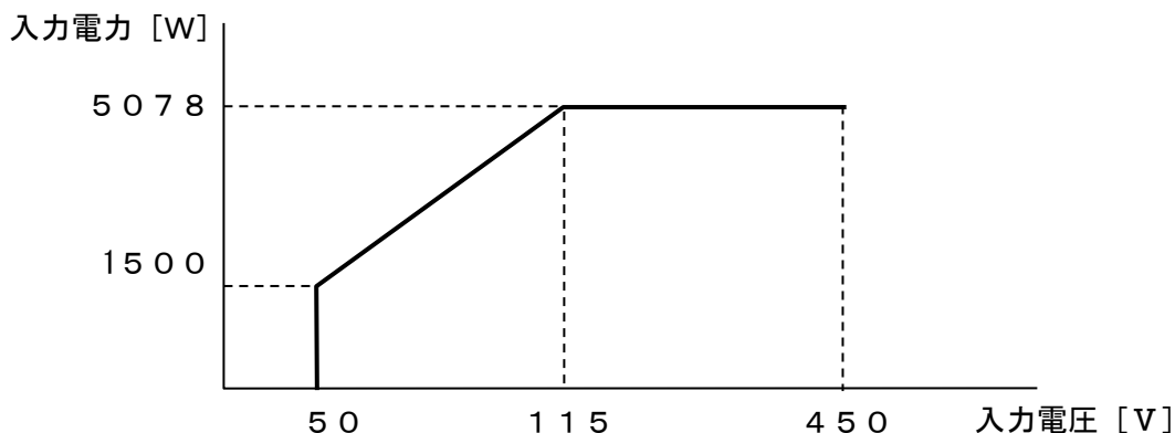
図3-1 直流入力電圧と入力電力との関係
