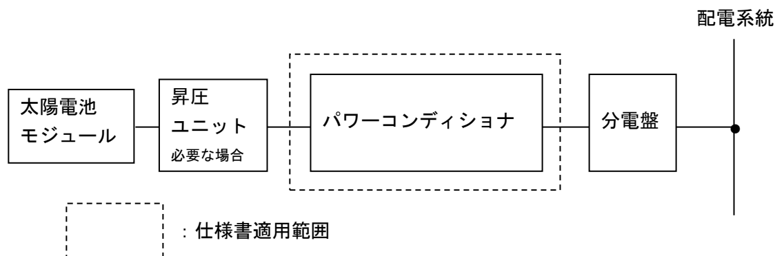
図2-1 全体構成図
