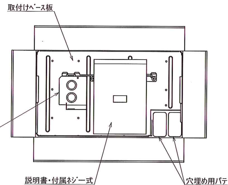
△B フソクビンケース梱包詳細図
