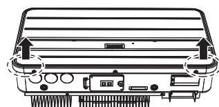
フロントカバー固定ねじ
