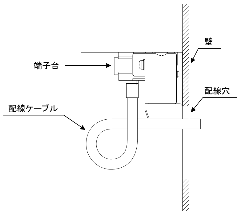
パワーコンディショナ右側面図
