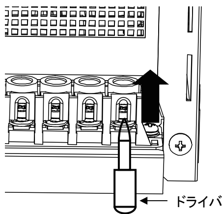
端子台付近の拡大図
