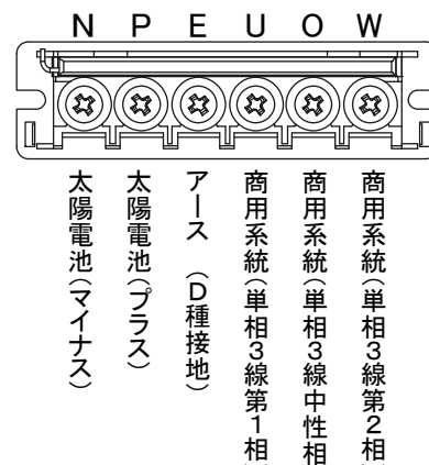
端子台の各端子の詳細
