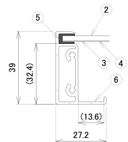
フレーム断面B-B'(1/2)
