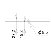
モジュール固定穴C(1/5)
